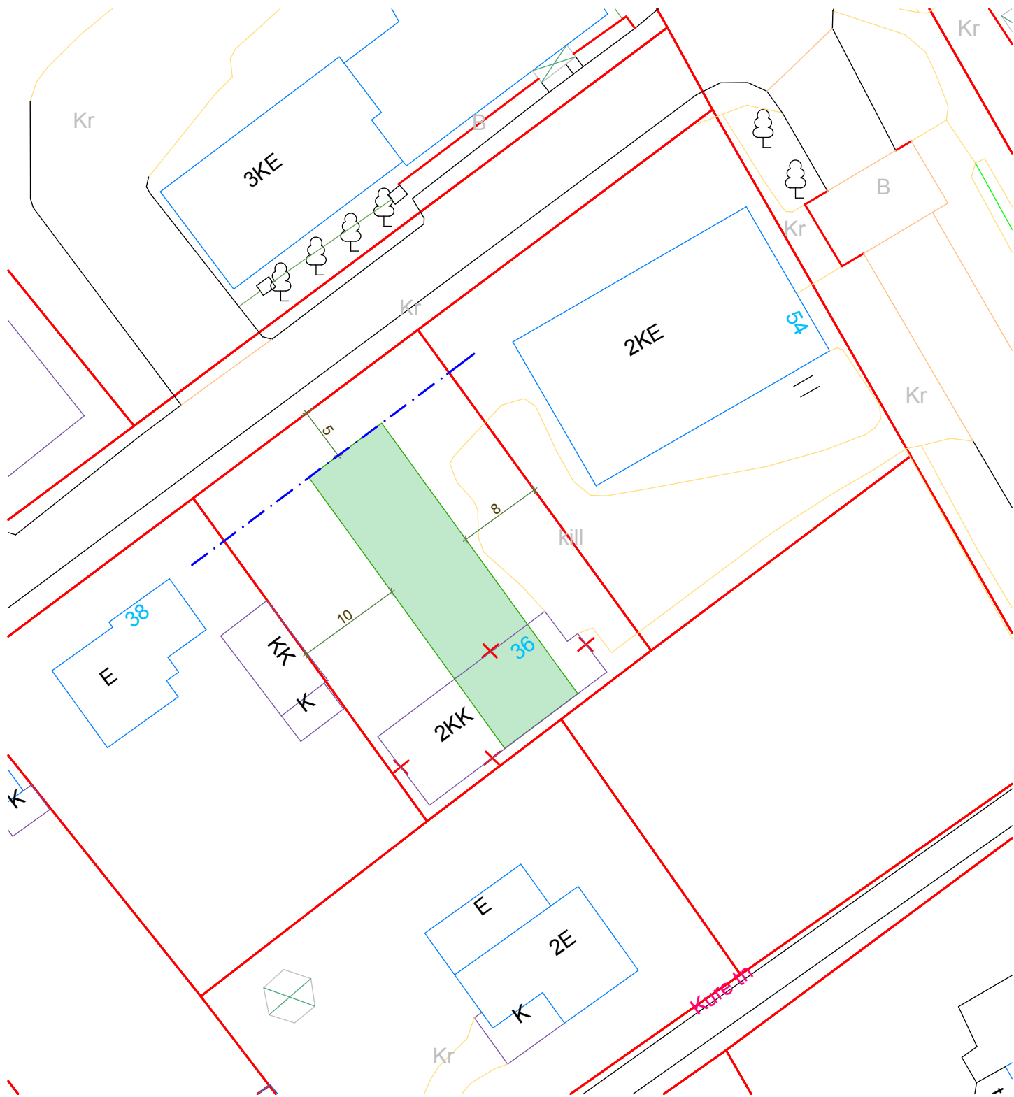
Lisa 1. Ehitusala skeem. PTH-16-031 Tamme pst 36
